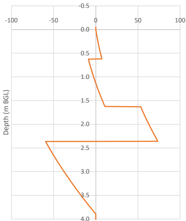
Shear (kN per end)
